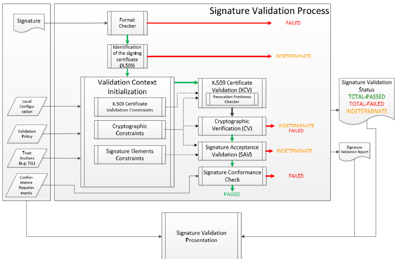
Ilustración 1 Basic Signature Validation ETSI TS 119 172-1
